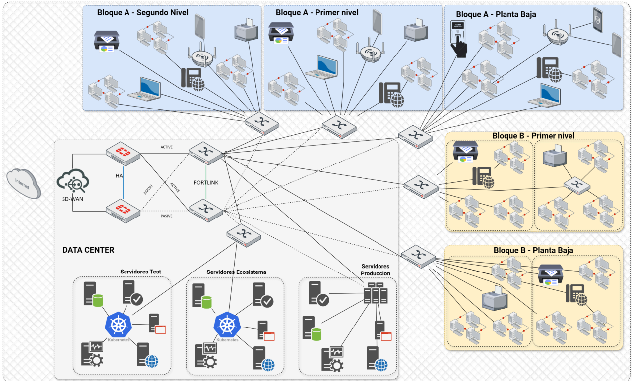
Diagrama de Red del Centro de Procesamiento de Datos de la Fiscalía General del Estado
