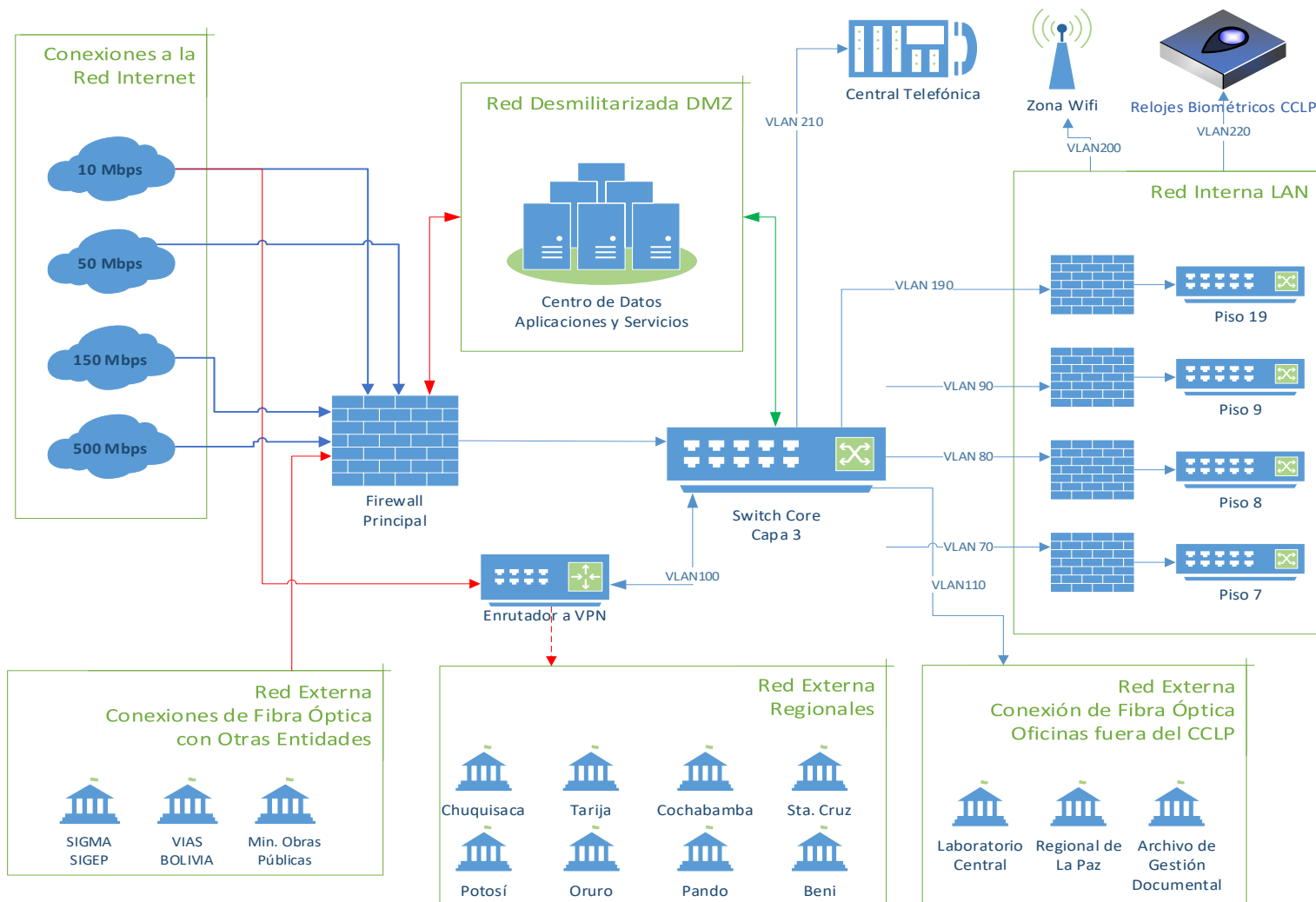
Imagen 3: Propuesta de RED para la ABC – Producto 2
