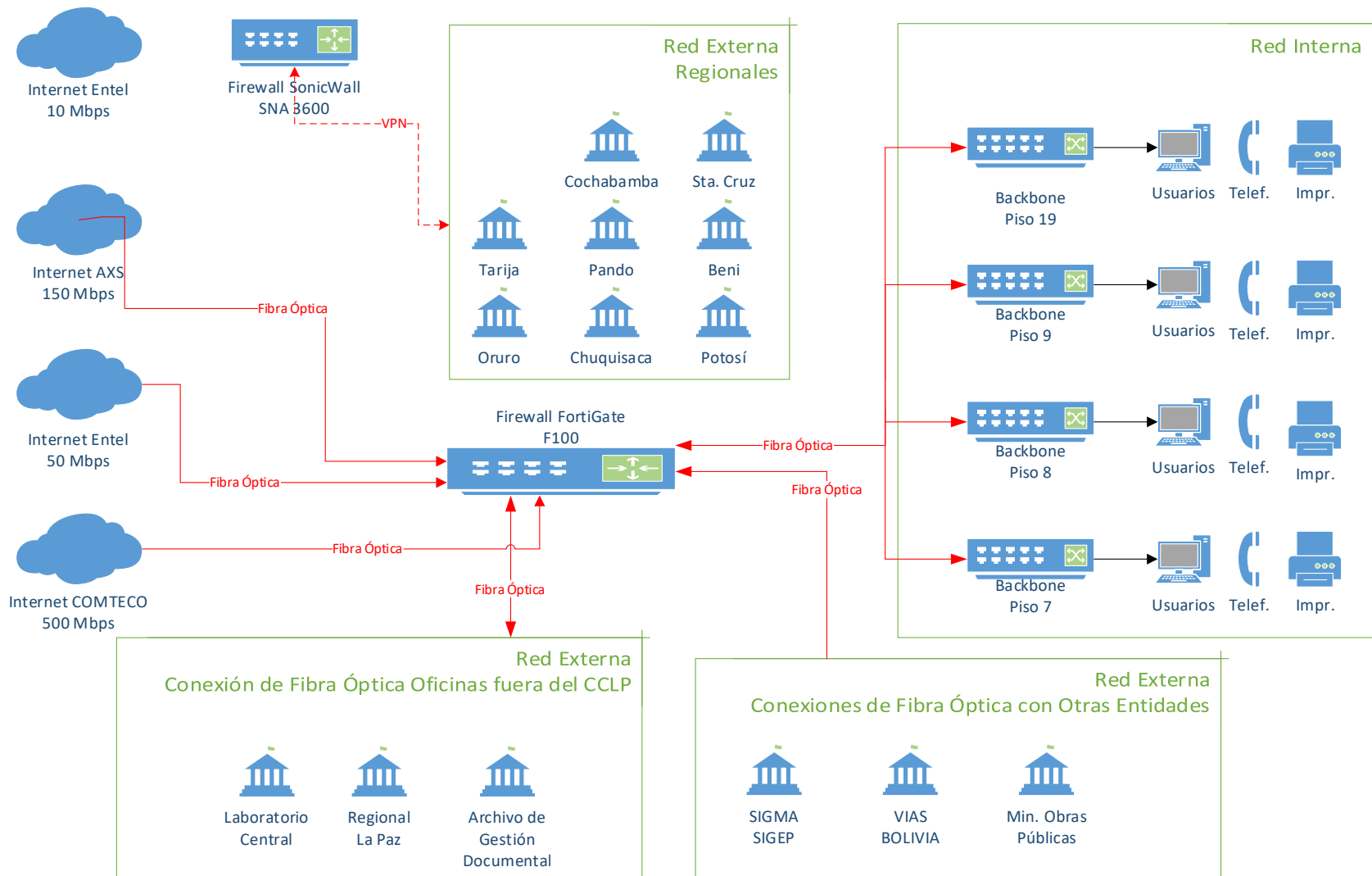
Imagen 1: Topología General de la Red de la Administradora Boliviana de Carreteras
